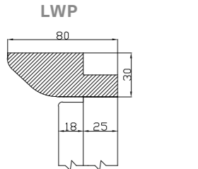
LISTWY PROSTE/ STRAIGHT CROWN MOULDINGS / GERADE KRONENLEISTEN
