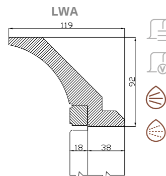
LISTWY PROSTE/ STRAIGHT CROWN MOULDINGS / GERADE KRONENLEISTEN
