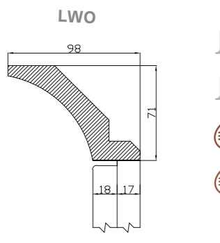
LISTWY PROSTE/ STRAIGHT CROWN MOULDINGS / GERADE KRONENLEISTEN
